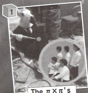
The \pi \times \pi 's
